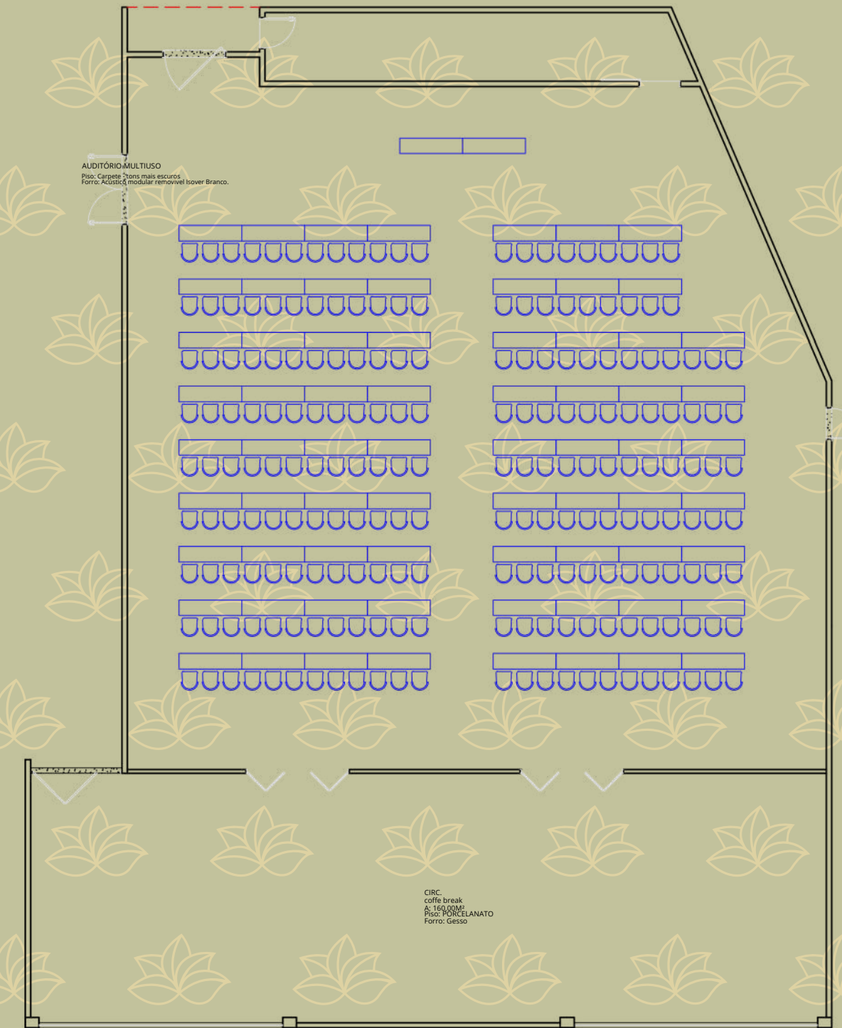
PLANTA LAYOUT AUDITÓRIO ESCOLAR - 210 PESSOAS
